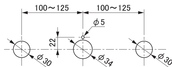
水栓金具取付穴
