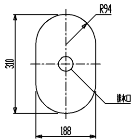
カウンター嵌込寸法
